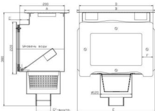
Рис. 1. Общий вид и габаритные размеры СК.30.0
