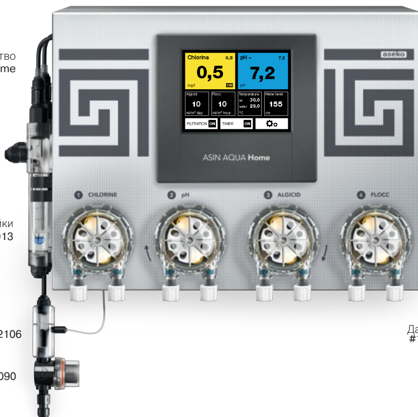
Перистальтические насосы #12093
