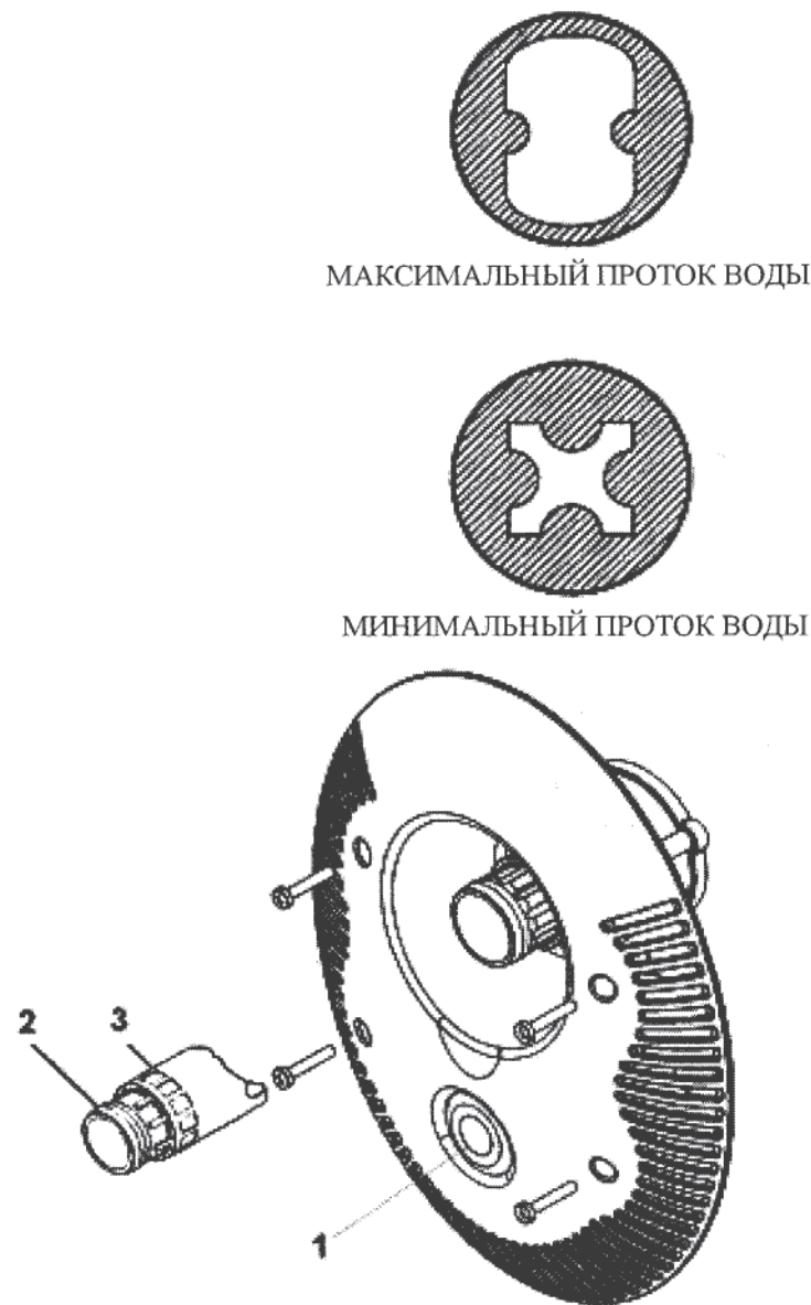
ИЗОБРАЖЕНИЕ ФОРСУНКИ ПРОТИВОТОКА
