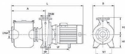
РАЗМЕРЫ
