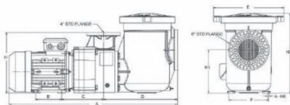
РАЗМЕРЫ
