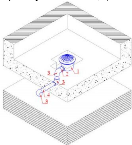
Рисунок 9 (установка сквозь дно)
