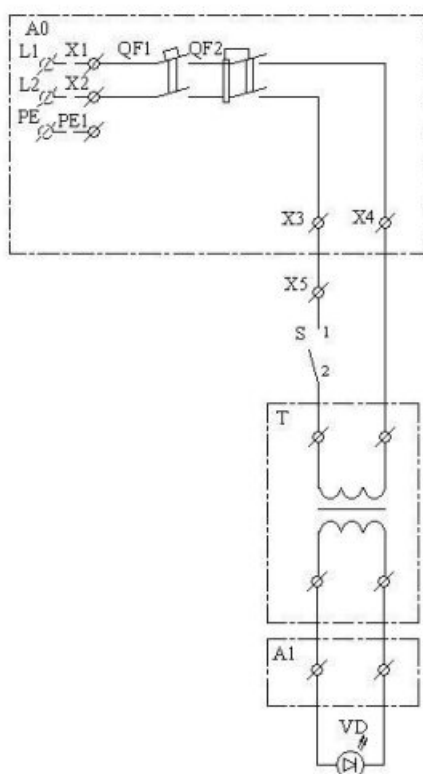
Электрическая схема 1
