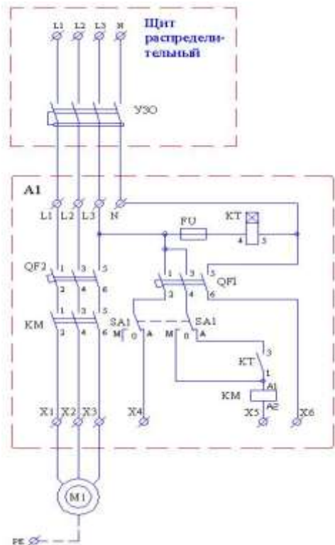
Эл.схема 1
