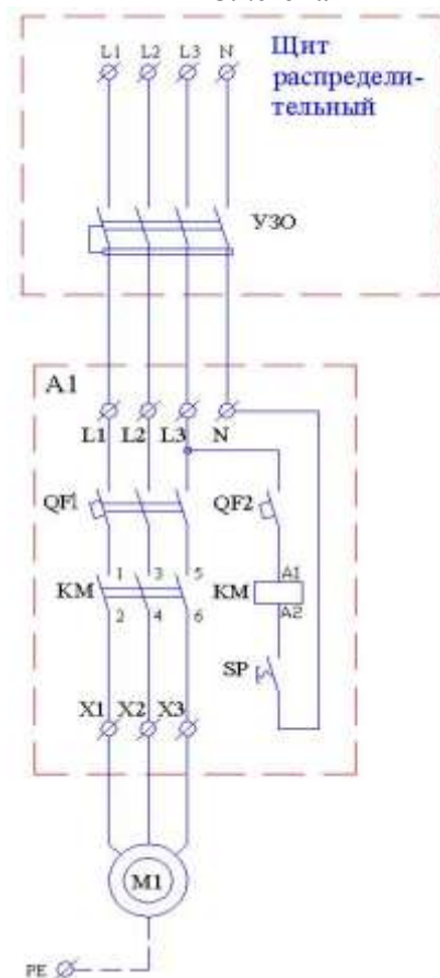
Эл.схема 2
