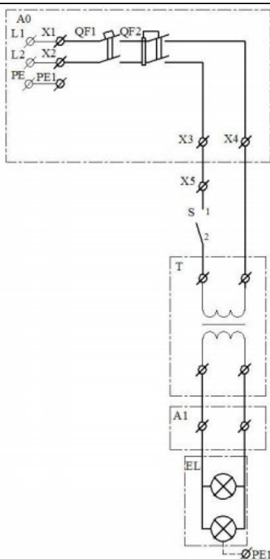
Электрическая схема 1
