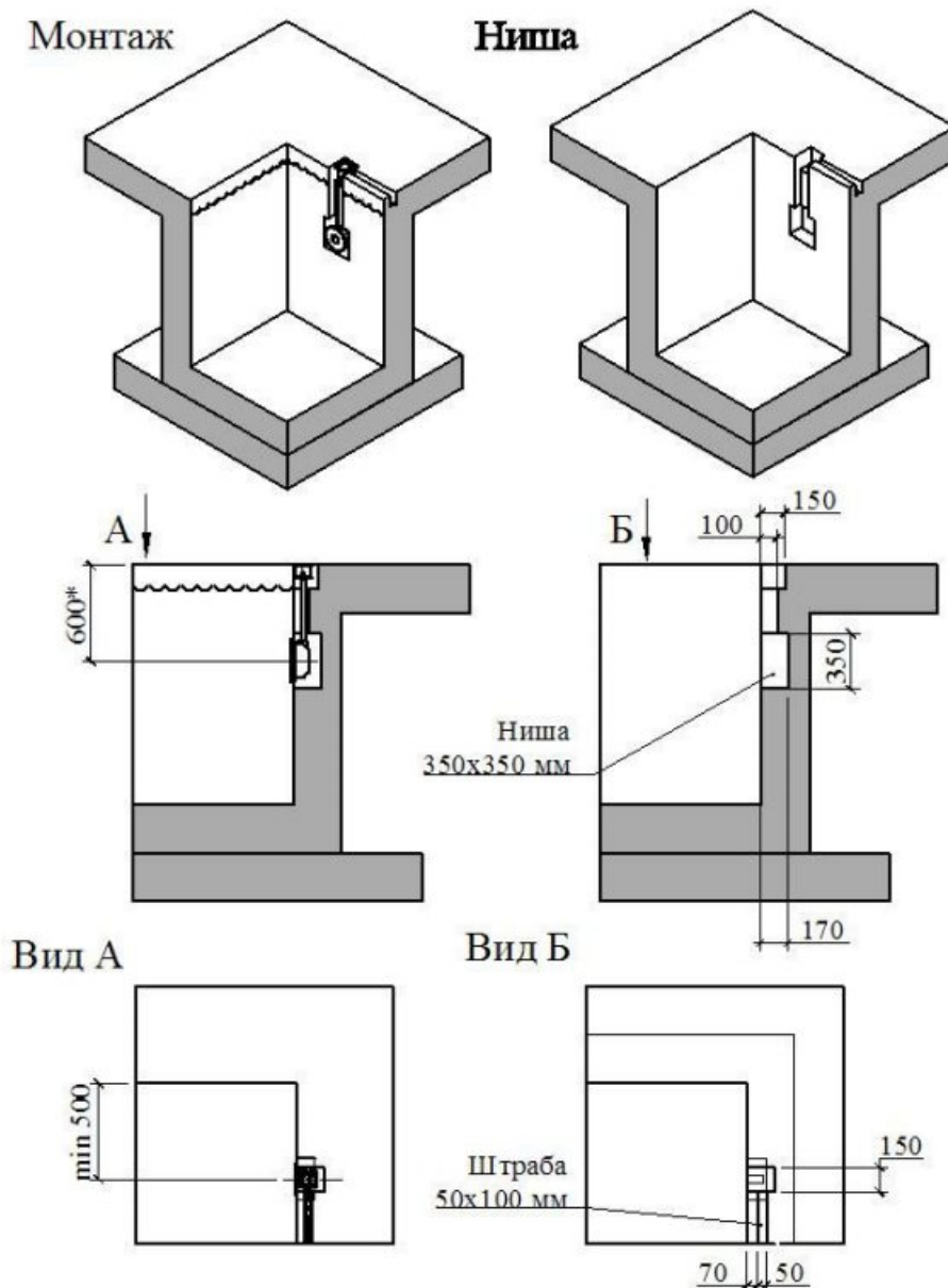
Рисунок 4 (Установка в переливной бассейн)
