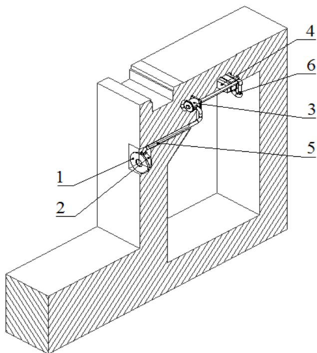
Рисунок 5 (Установка в скиммерный бассейн)
