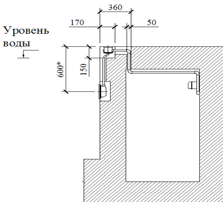
Рисунок 8 (Установка в скиммерный бассейн)
