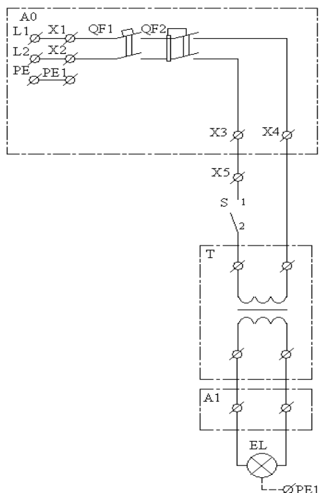
Электрическая схема 1
