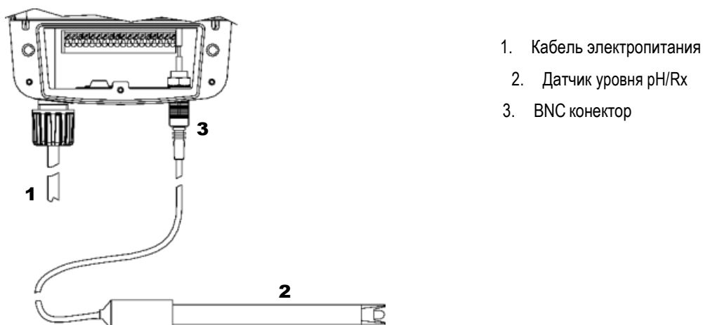
Fig. 10 – Подсоединение датчика pH или REDOX
