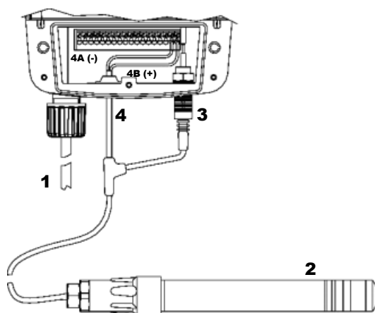
Fig. 11 – Подсоединение датчиков CI и PPM
