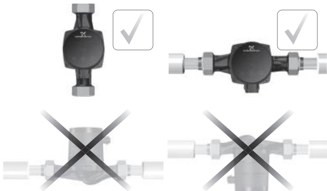
Рис. 5 Расположение насоса
