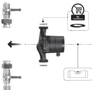
Рис. 3 Монтаж насоса
