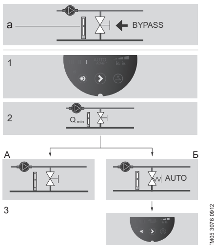
Рис. 18 Системы с перепускным клапаном
