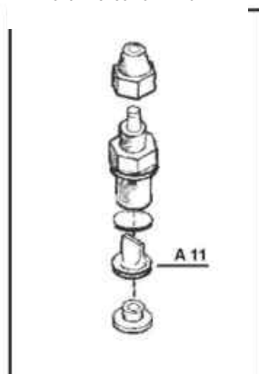
Клапан лепестковый 20 л/ч
