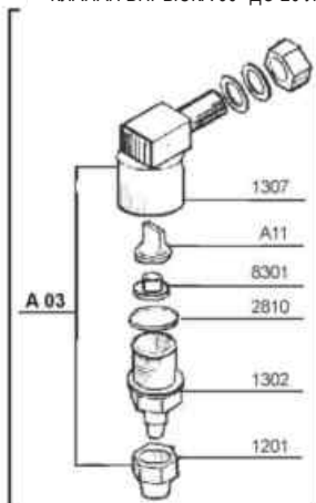
КЛАПАН ВПРЫСКА 90° ДО 20 Л/Ч
