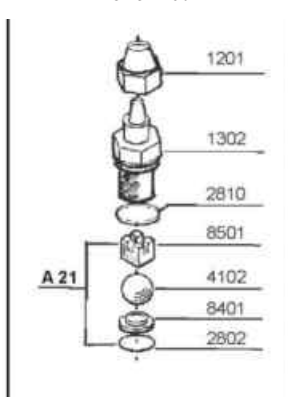
КЛАПАН ОБРАТНЫЙ САМОТЕЧНЫЙ ШАРОВОЙ 20 Л/Ч
