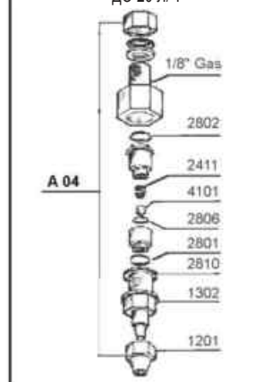
КЛАПАН ВПРЫСКА ШАРОВОЙ ДО 20 Л/Ч
