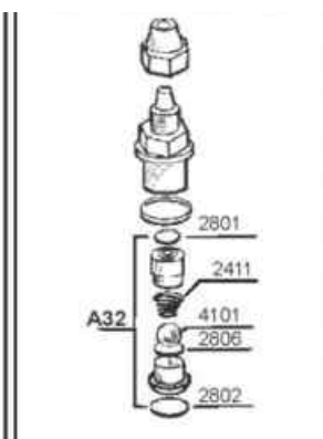
КЛАПАН ВЫПУСКНОЙ ОБРАТНЫЙ ШАРОВОЙ
