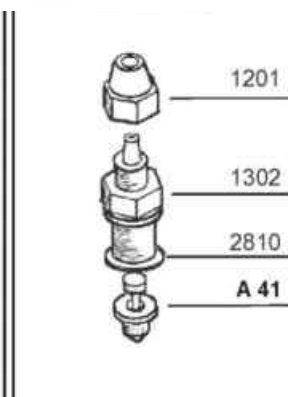
КЛАПАН ТИПА KALRETZ
