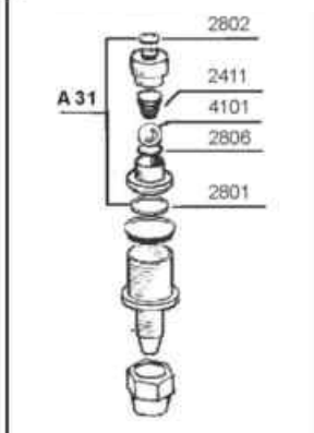
КЛАПАН ВСАСЫВАЮЩИЙ ОБРАТНЫЙ ШАРОВОЙ
