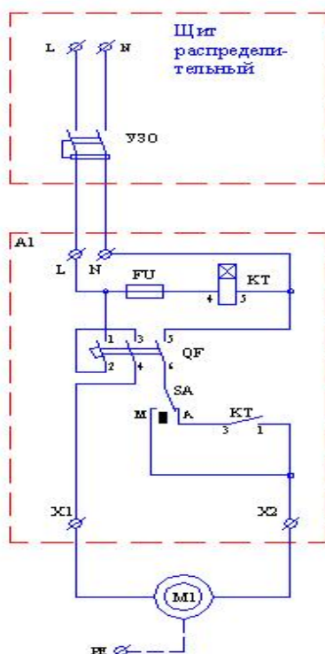
Эл.схема 1
