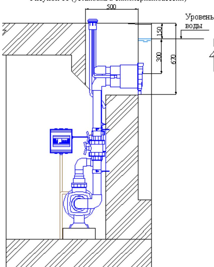
Рисунок 11 (установка в скиммерный бассейн)
