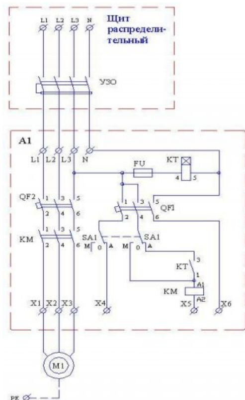
Эл.схема 1
