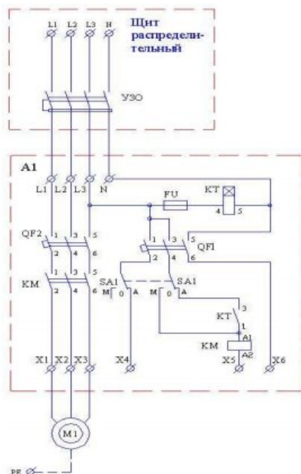
Эл.схема 1
