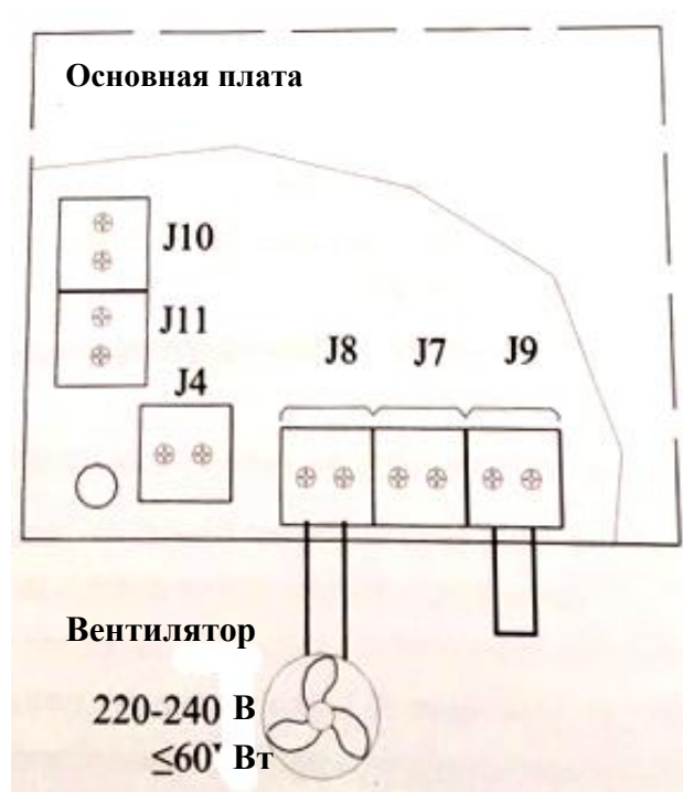
Рисунок 19 Схема подключения вентилятора
