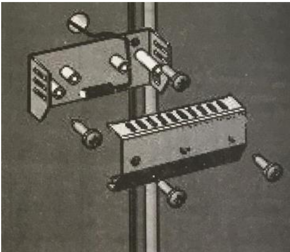
Рисунок 17 Установка датчика температуры
