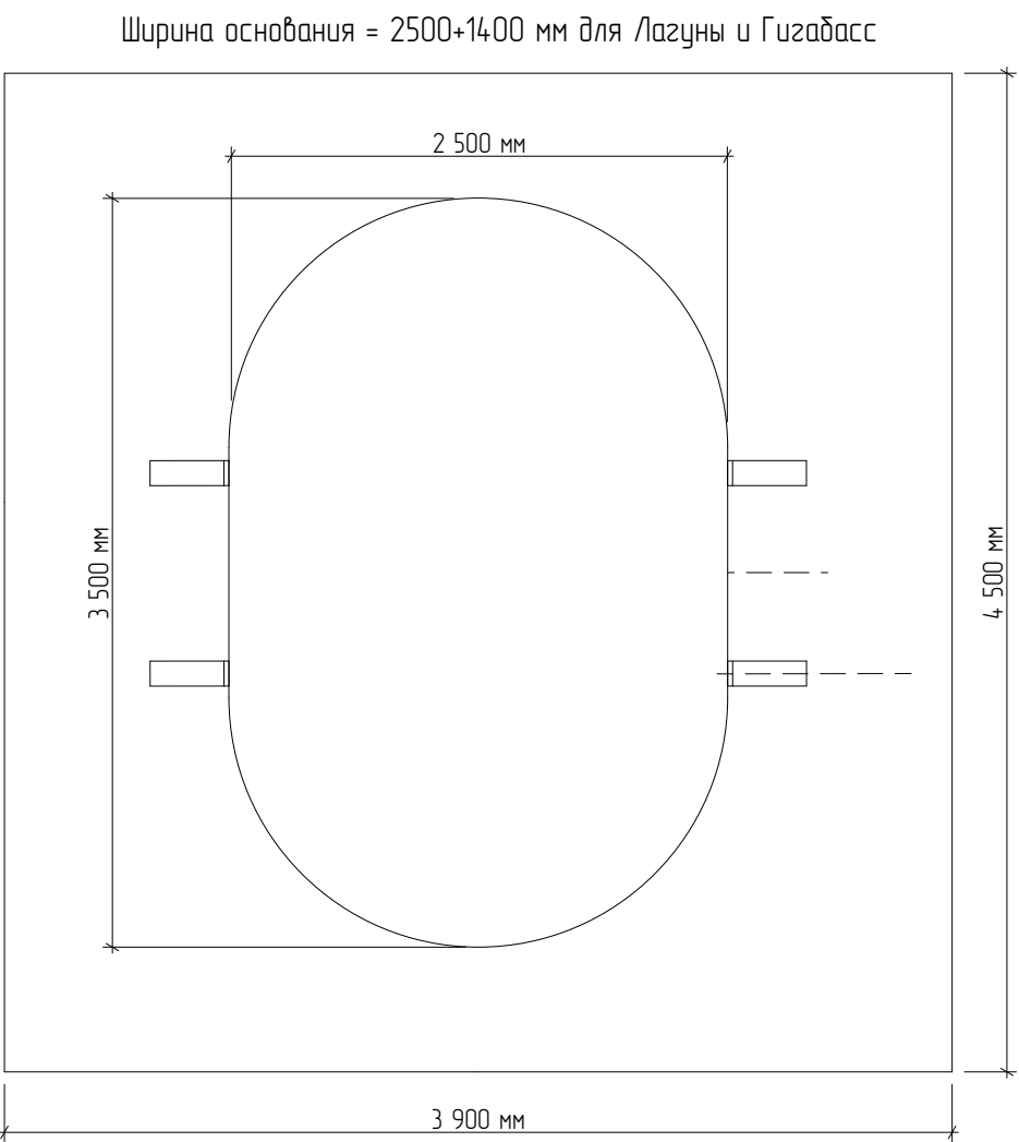
Вид сверху
