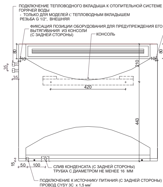
ВИД СНИЗУ
