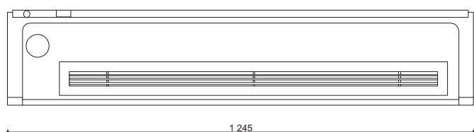
ВИД СНИЗУ
