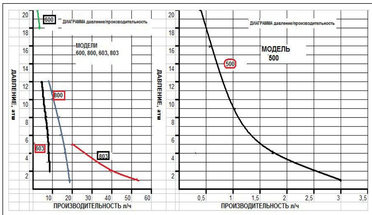
Рисунок 1. Диаграмма рабочих характеристик насосов-дозаторов
