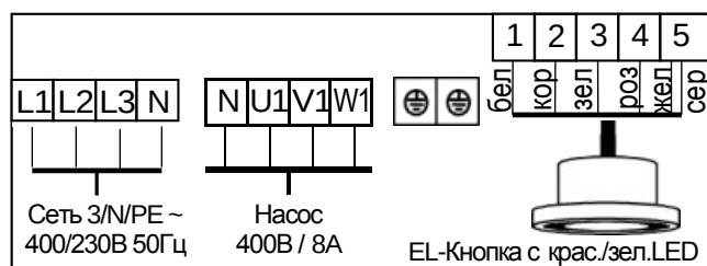
Подключение трехфазного насоса 400В
