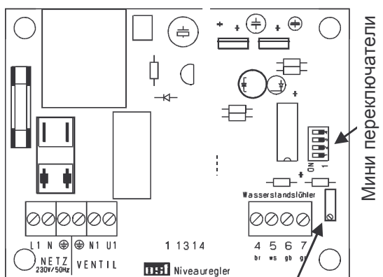
Регулировочный потенциометр
