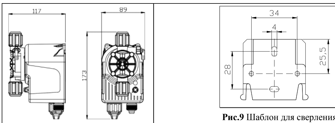
Рис.8 Габаритные размеры
