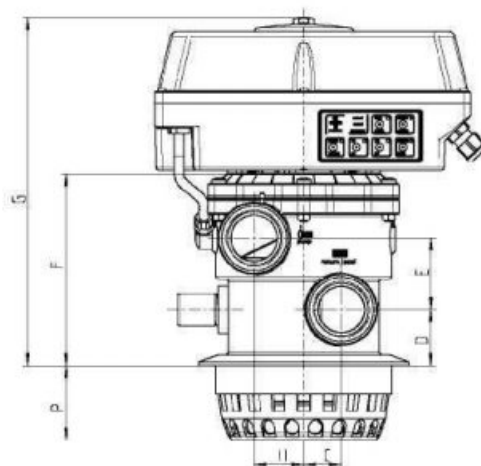
Вертикальный монтаж
