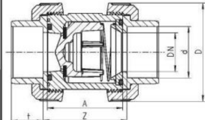
Запорный клапан S6
