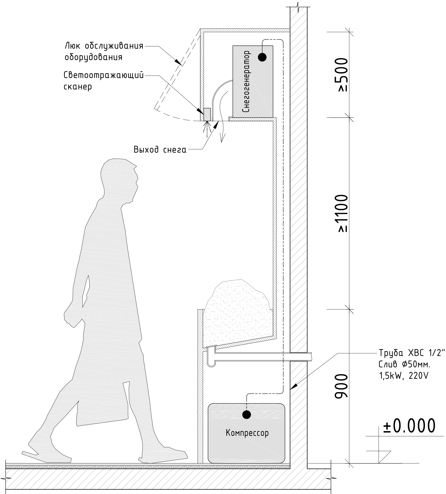
Вариант А Сплит-система
