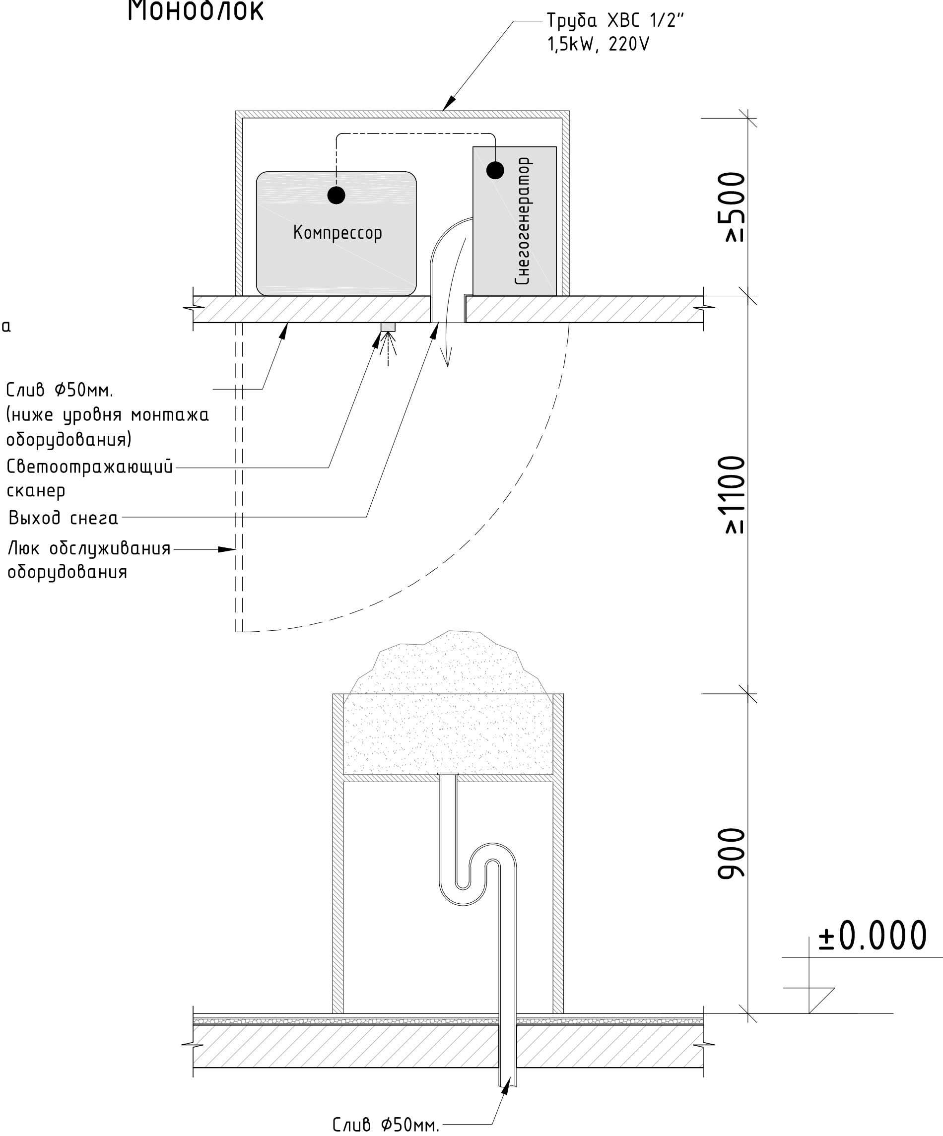
Вариант D Моноблок
