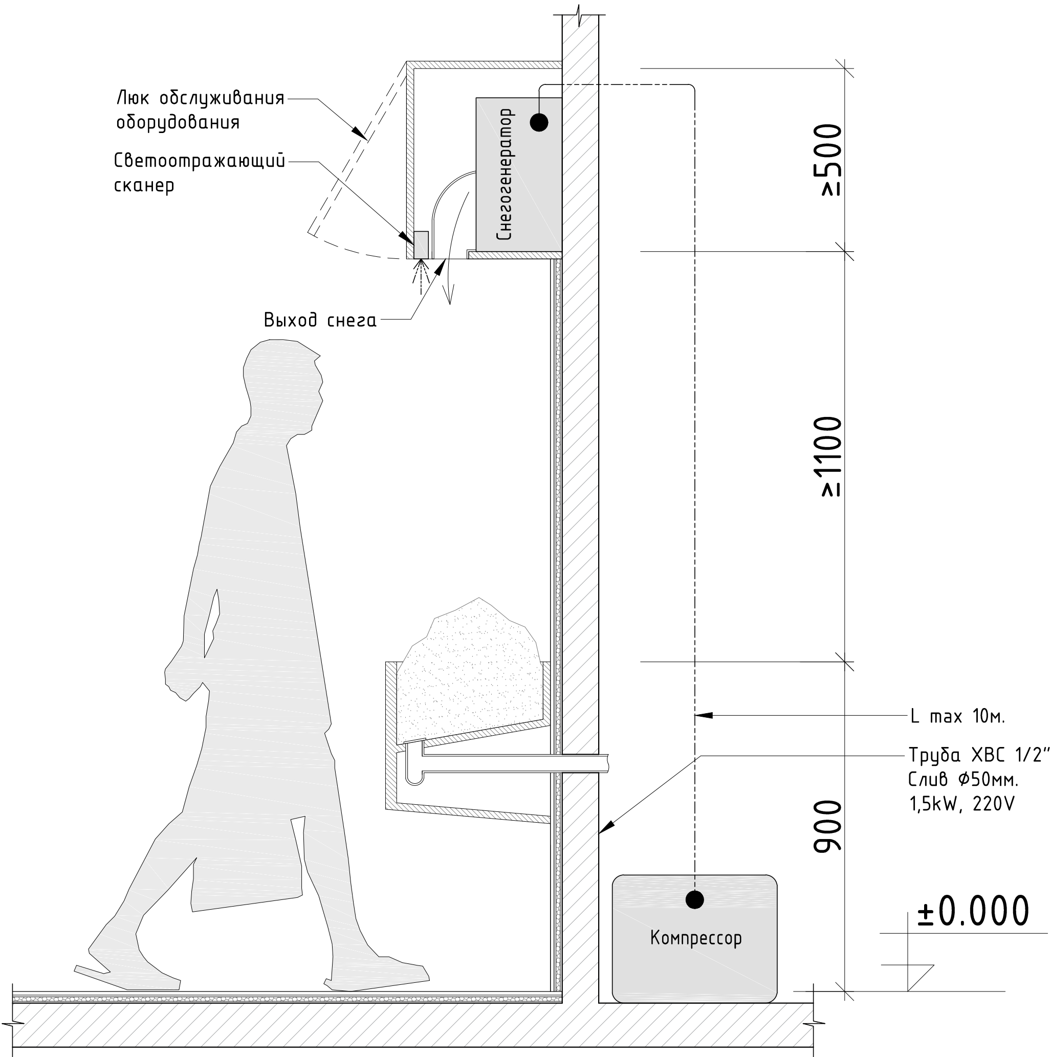
Вариант В Сплит-система
