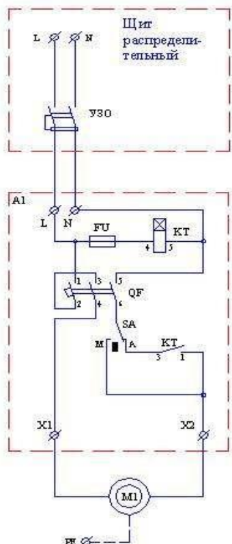
Эл.схема 1
