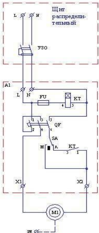
Эл.схема 1
