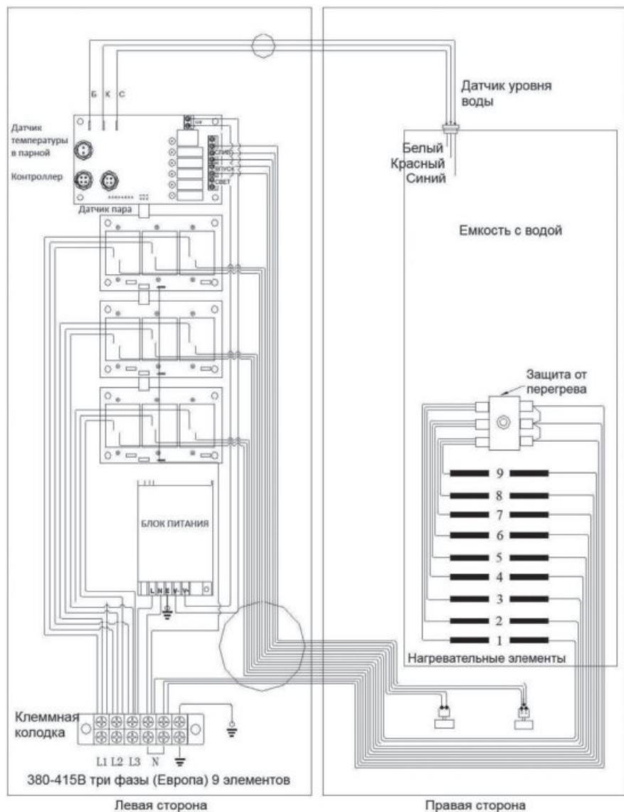
Рисунок 12. Электромонтажная схема TOLO-150 KEY - TOLO-240 KEY
