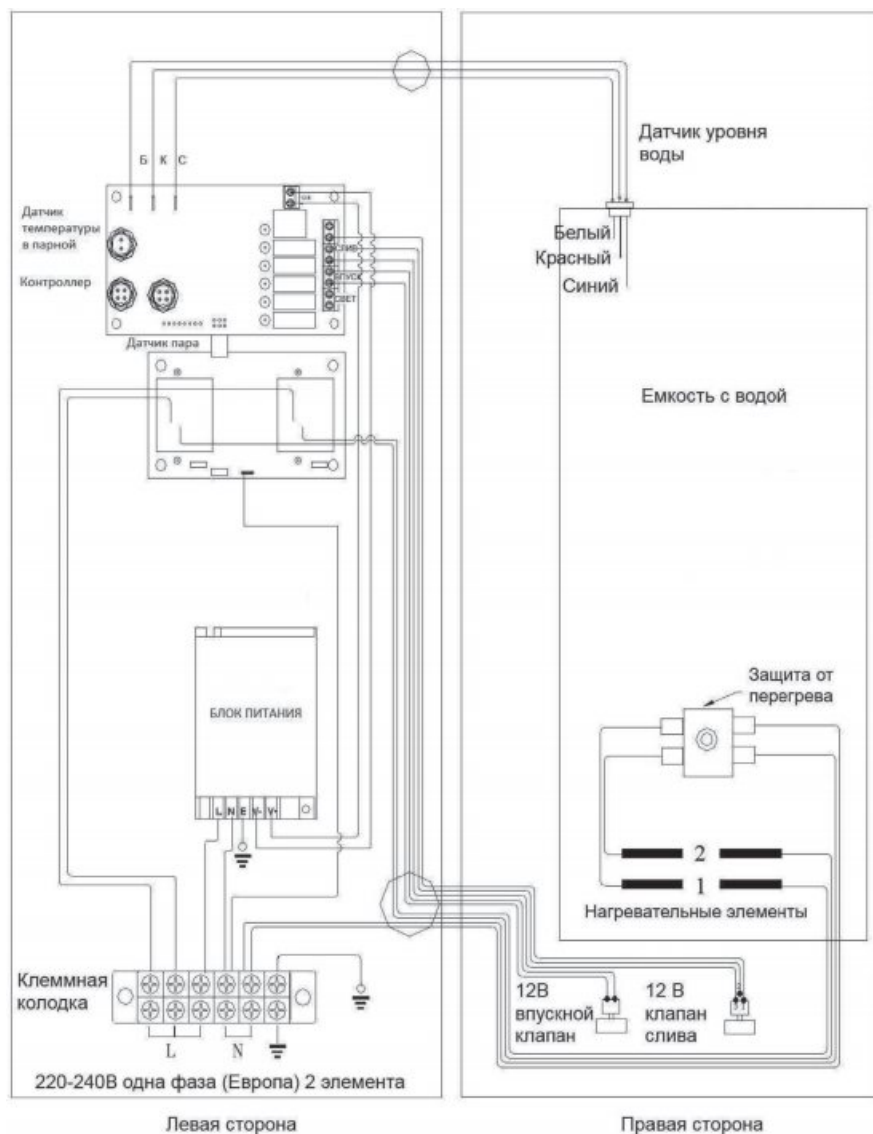
Рисунок 9. Электромонтажная схема TOLO-30 KEY
