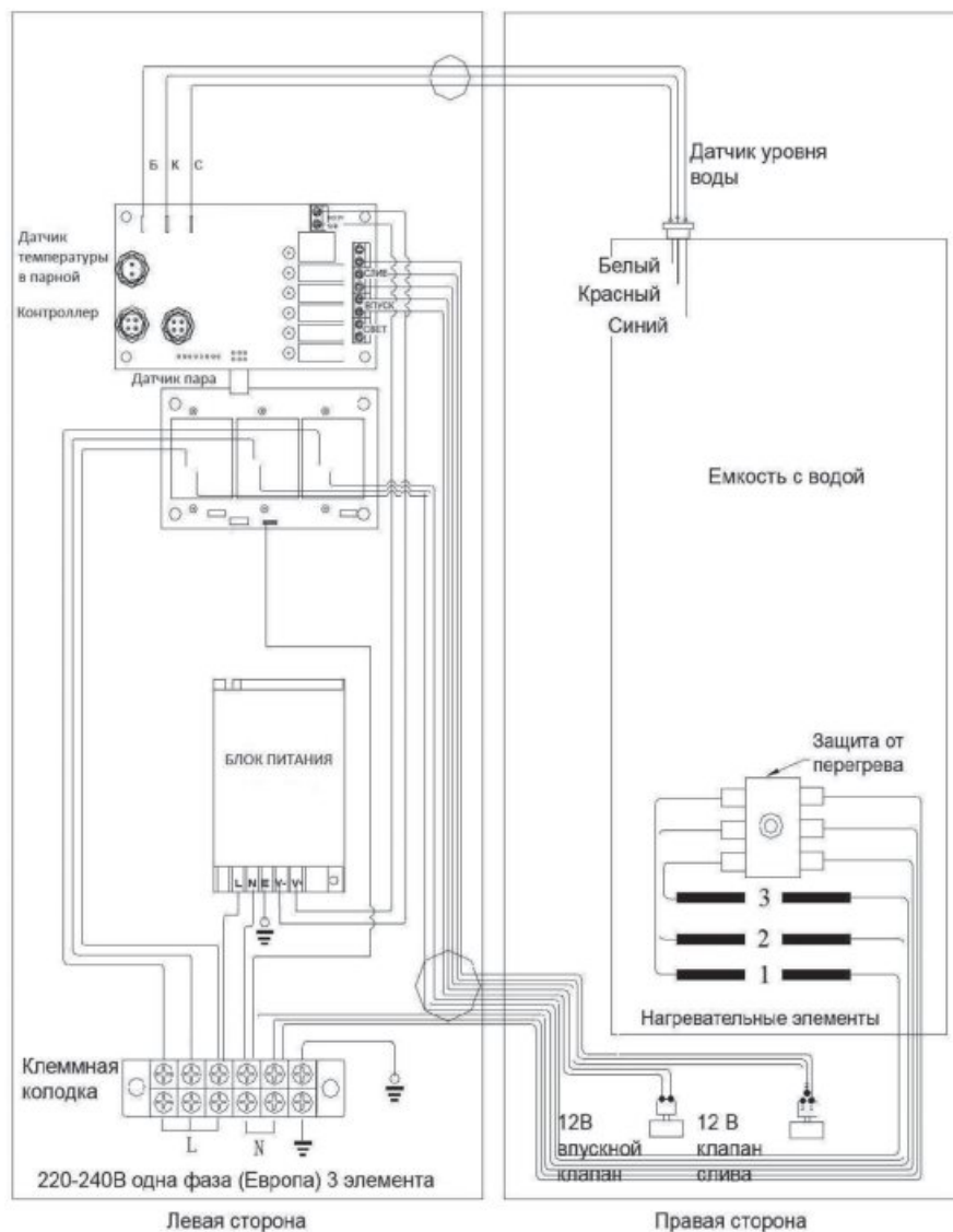
Рисунок 10. Электромонтажная схема TOLO-40 KEY - TOLO-80 KEY
