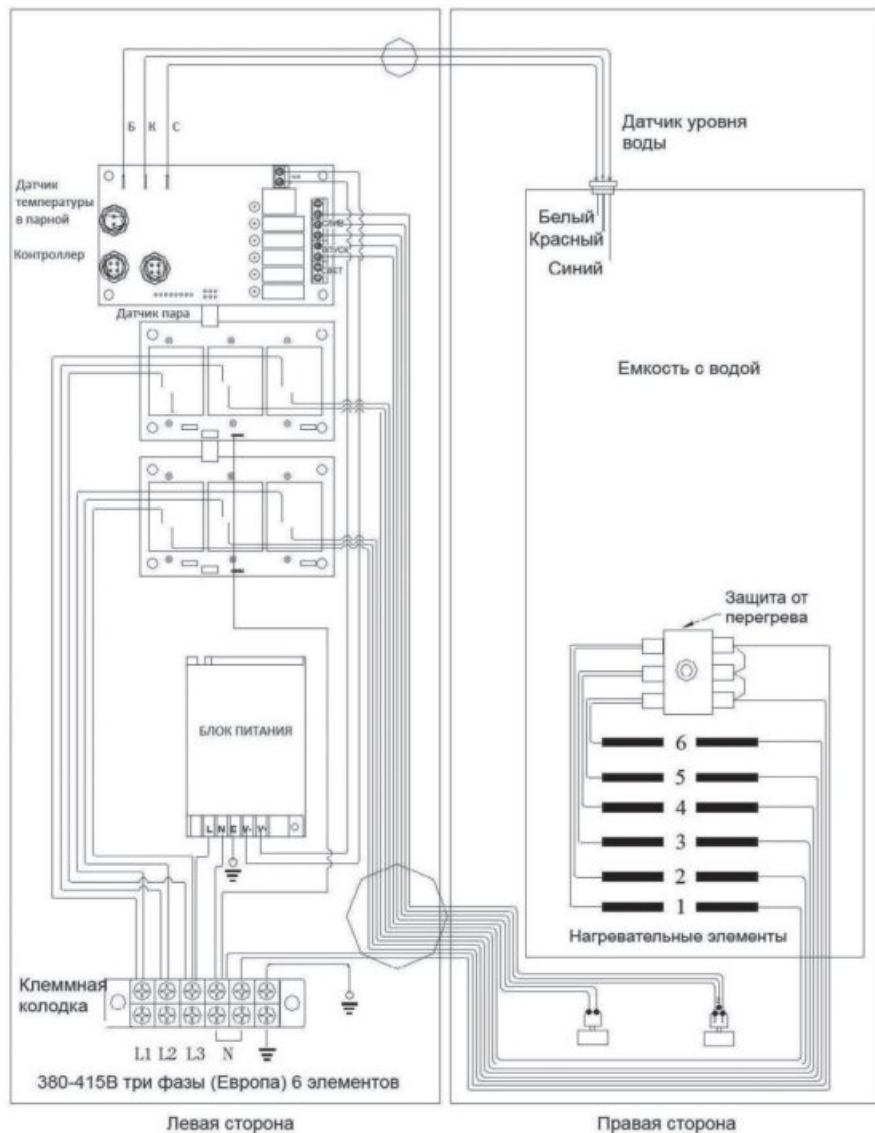
Рисунок 11. Электромонтажная схема TOLO-90 KEY - TOLO-135 KEY
