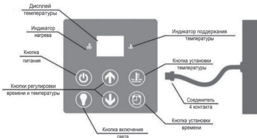
Рисунок 3. Панель управления
