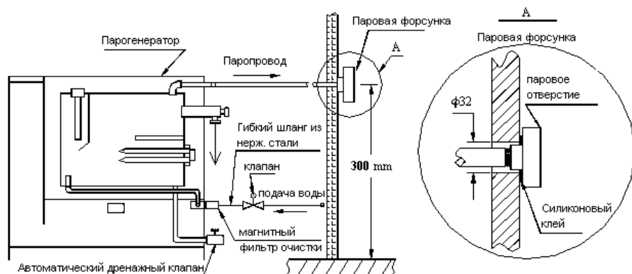
Рисунок 7. Схема подключения
