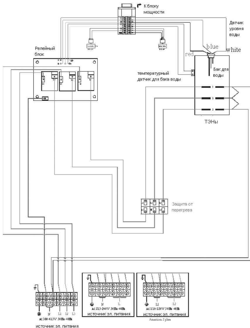
Рисунок 8. Электромонтажная схема для пультов AIO-30, AIO-40, AIO-60, AIO-75
