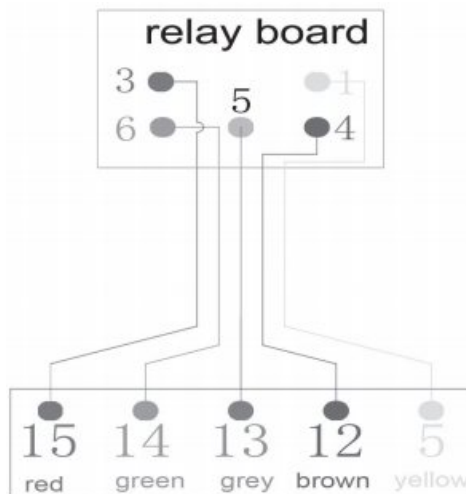
Рисунок 13. Описание последовательности линии VGA реле в парогенераторе
