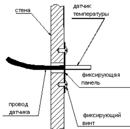
Рисунок 6. Установка датчика температуры
