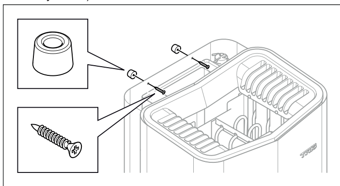
Рис 12: Разместите шайбы
