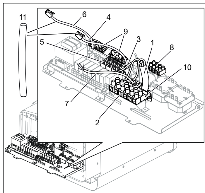
Рисунок 10: Монтажная плата
