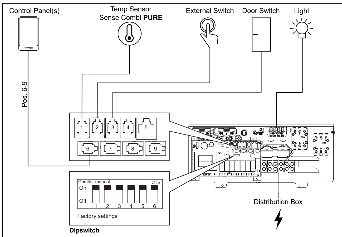
Рис. 20. Схема установки Sense Combi Pure
