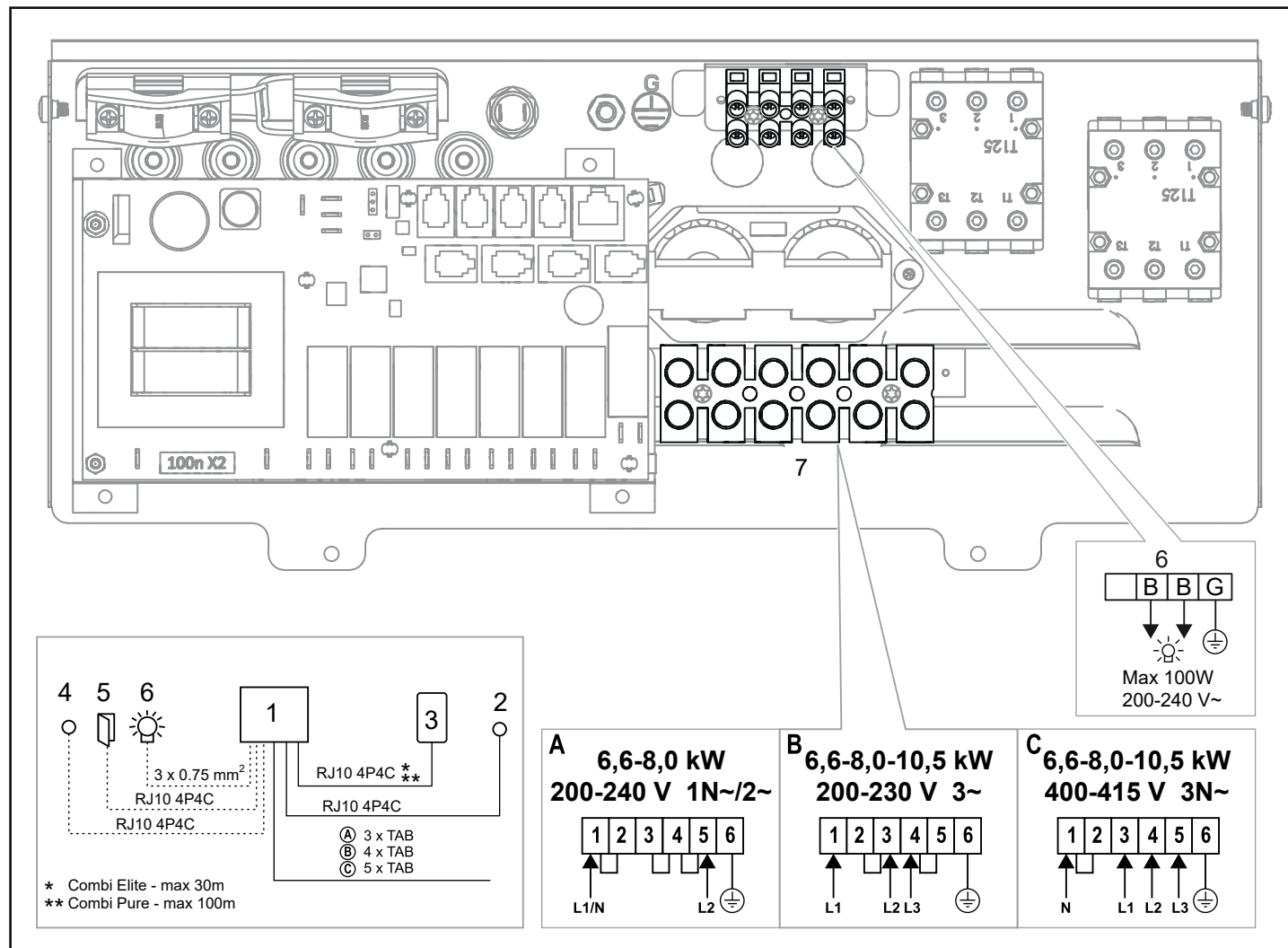
Рисунок 17: Схема соединений
