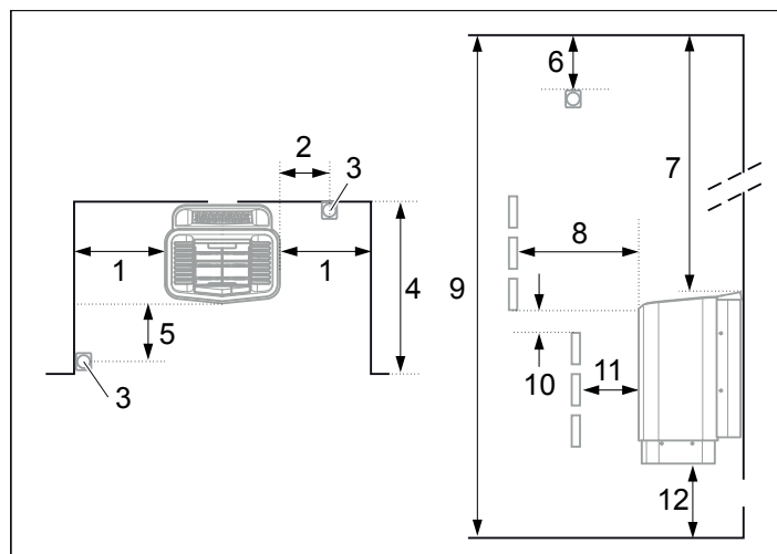
Рисунок 5: Позиционирование нагревателя - установка в нише
