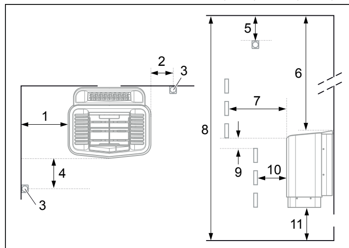
Рисунок 3: Позиционирование нагревателя - нормальная установка
