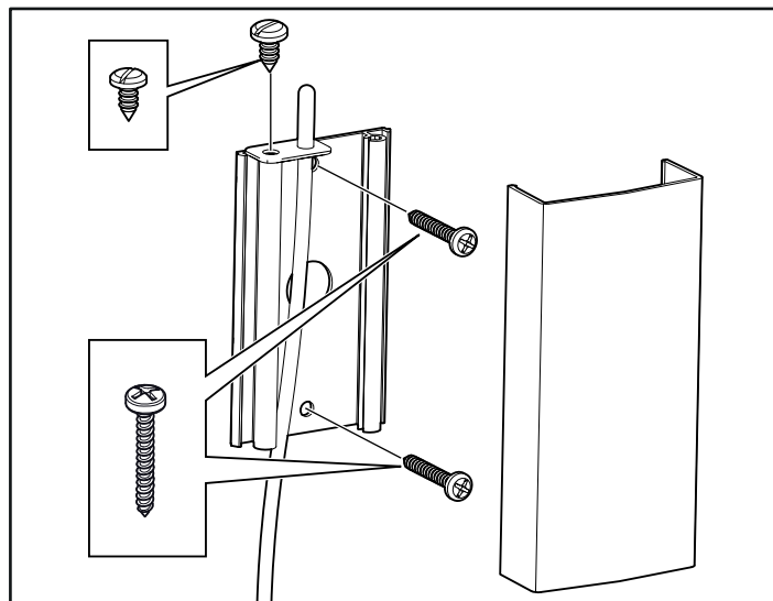
Рисунок 21: Установка датчика
