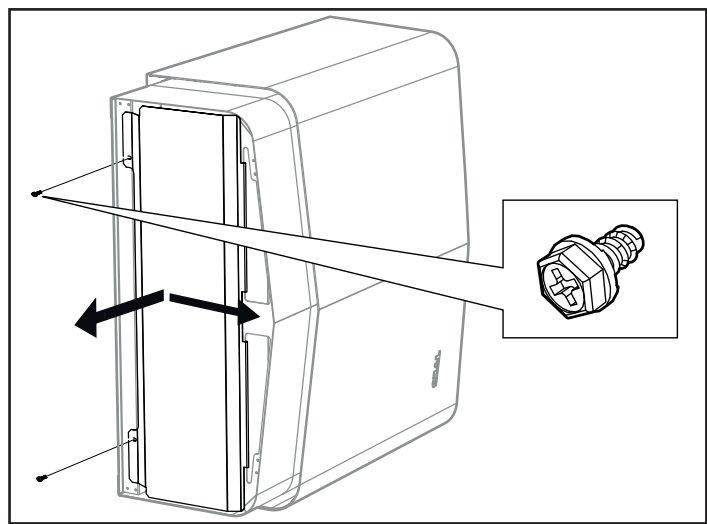
Рисунок 15: Открытие/закрытие крышки
