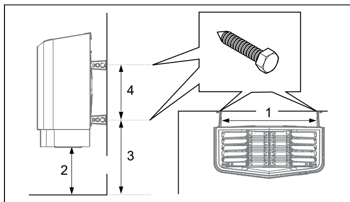
Рисунок 18: Размеры
