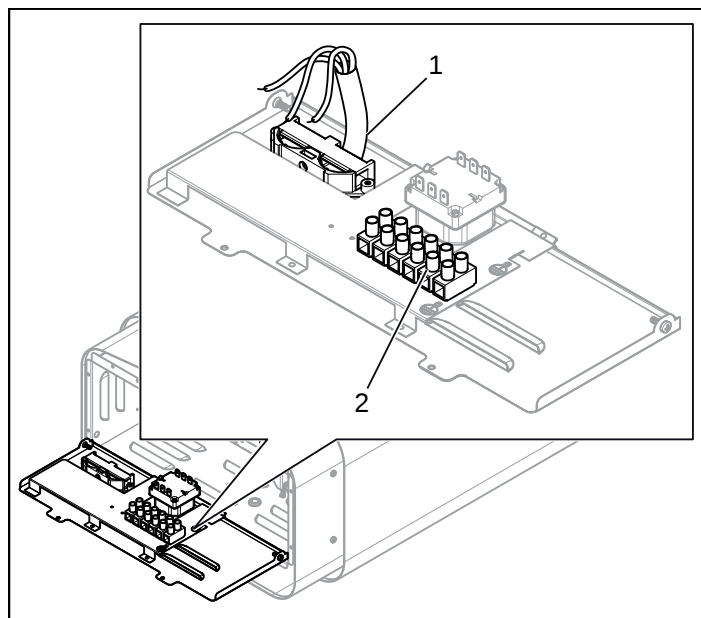
Рисунок 11: Электрическое соединение
