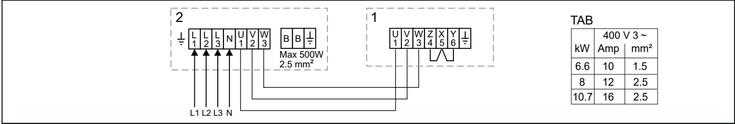
Рисунок 31: Панель управления TS 16-6B
