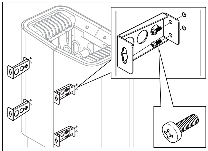
Рисунок 12: Крепление кронштейнов к нагревателю
