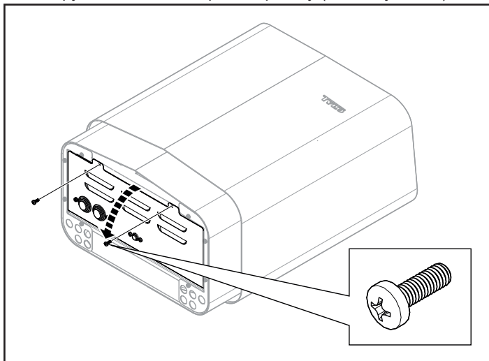
Рисунок 10: Открытие/закрытие крышки
