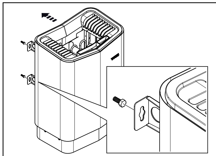
Рисунок 19: Навесьте нагреватель.
