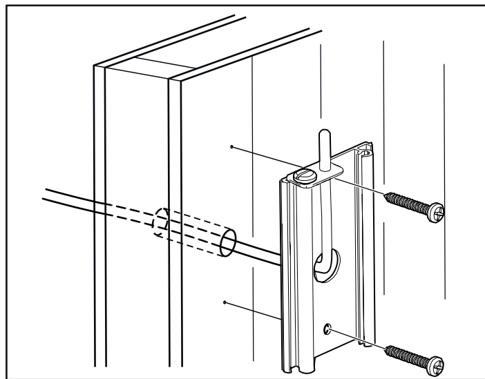
Рисунок 22: Проведение проводки через стену.
