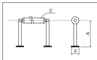
Телескопическое наматывающее непередвижное устройство с электрическим приводом
