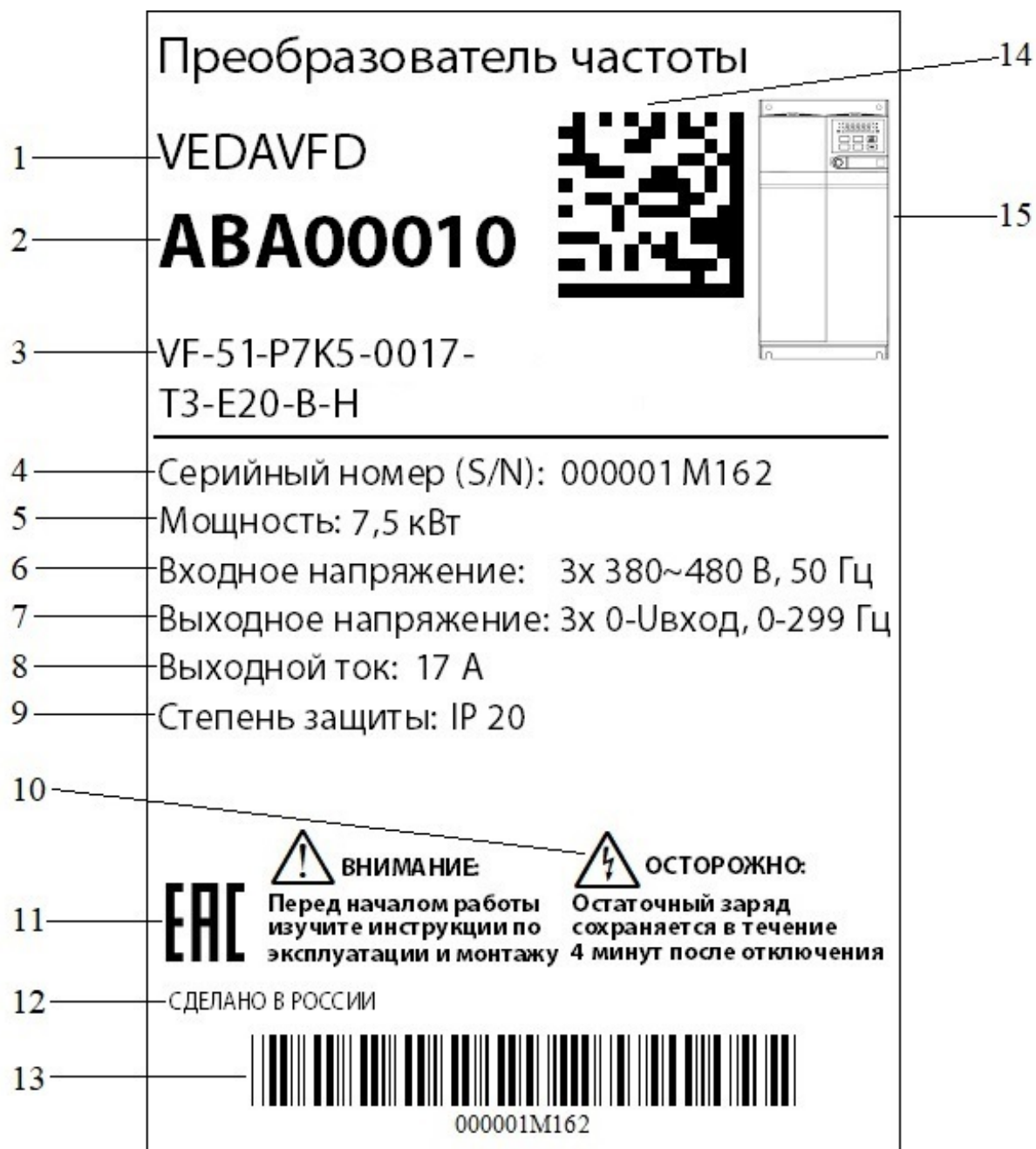
Рис. 1-3. Пример маркировки преобразователя частоты
